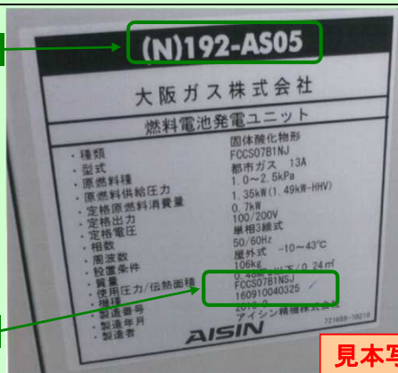
②燃料電池ユニットの品名・製造番号のアップ
